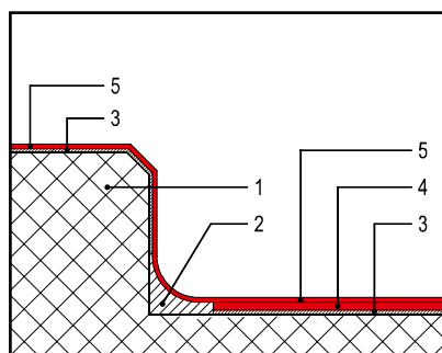
Raccords courbes rigides avec raccordement à la maçonnerie
